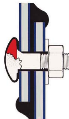
Verschraubung / Eindichtung der Segmentplatten
