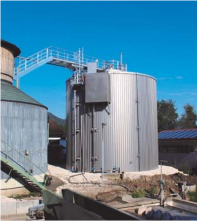
Piding, Baujahr 2014 Faulbehälter 740m 3 Besonderheit: Schlammtasche Werkstoff: V4A
